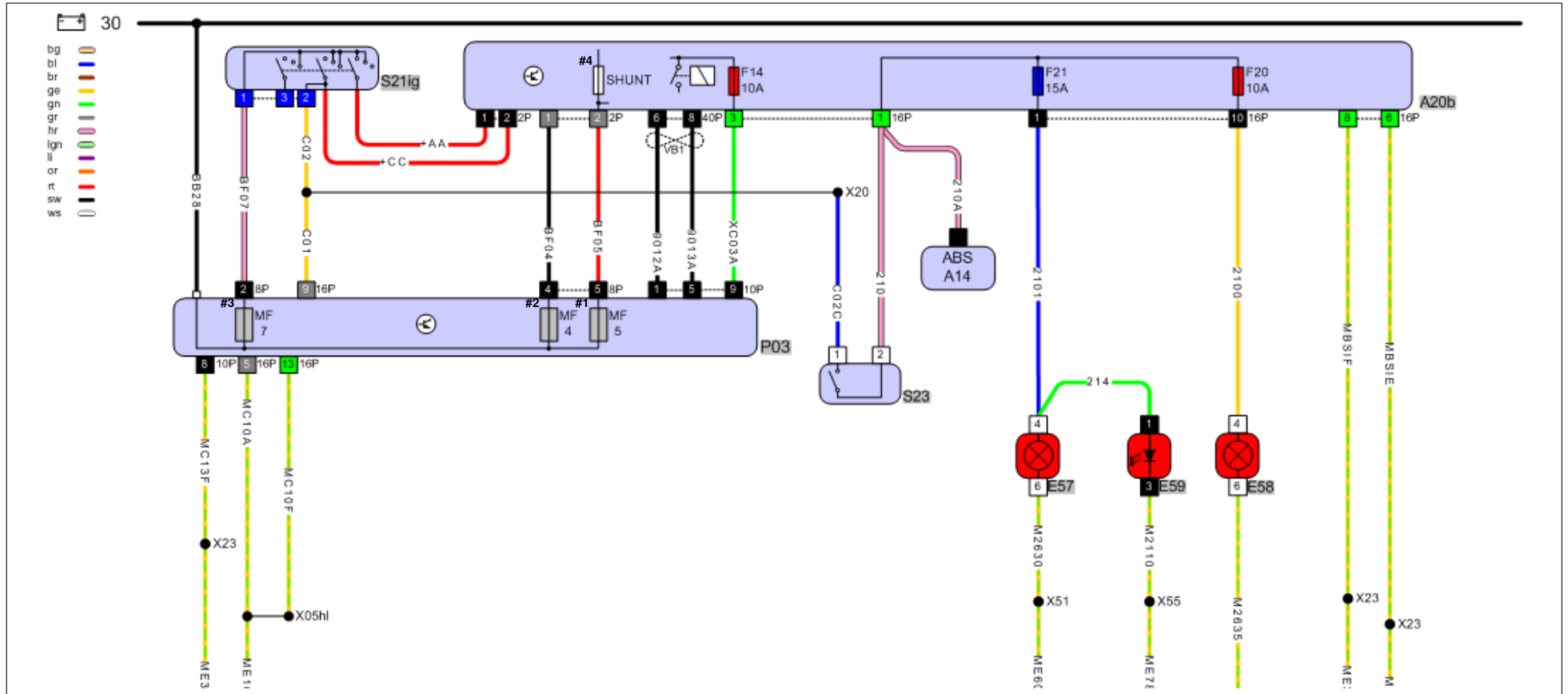
Abbildung 2: Zusatz &gt; Außenbeleuchtung &gt; Bremslicht &gt; 2002-11-04 - ... (vergrößerter Bildausschnitt)
