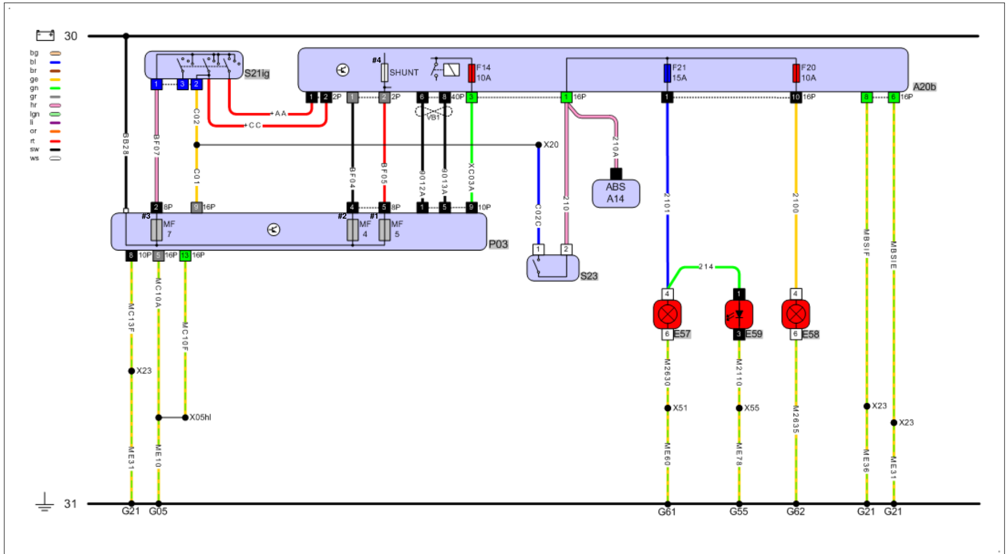
Abbildung 1: Zusatz &gt; Außenbeleuchtung &gt; Bremslicht &gt; 2002-11-04 - ... (Gesamtdarstellung)
