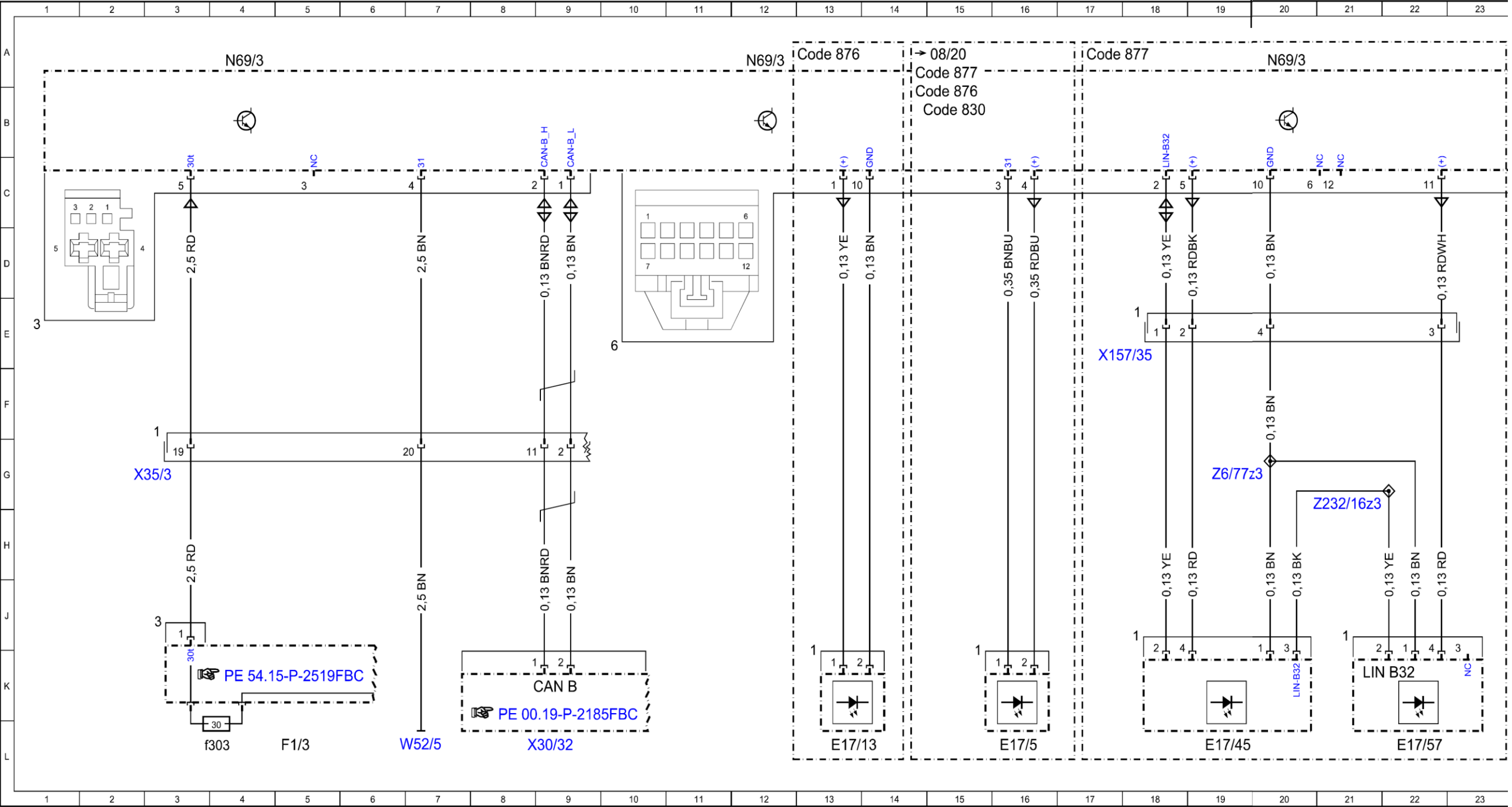
Documento: schema elettrico centralina porta posteriore sinistra
