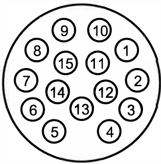
Stecker 15 polig
