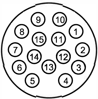
Connecteur 15 pôles
